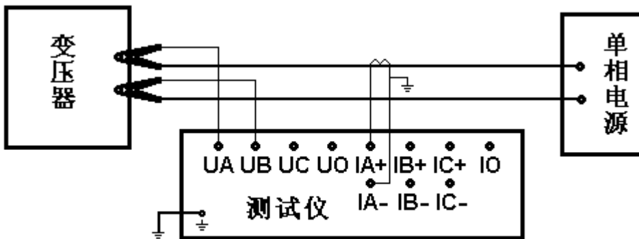
图 7-13 单相外接电流互感器接线图
