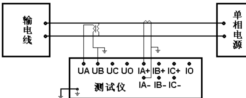
图 4-8 单相外接电压互感器和电流互感器接线图
