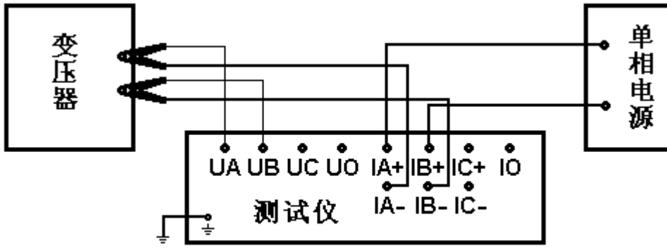
图 7-11 单相变压器直接测量接线图
