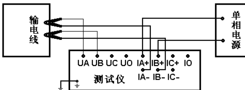
图 4-7 单相直接测量接线图
