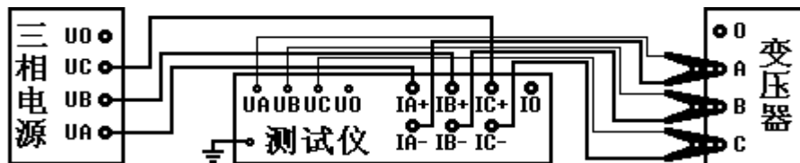
图 9-5 变压器容量分析接线图
