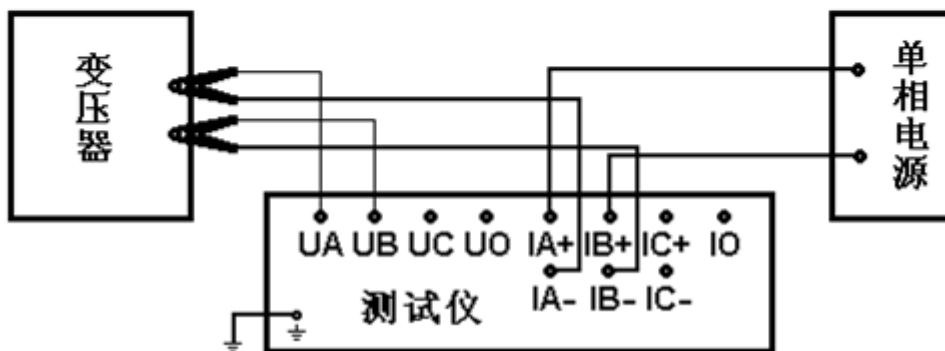
图 8-5 单相变压器直接测量接线图
