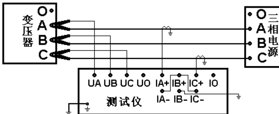
图 7-10 三相三线外接电流互感器接线图
