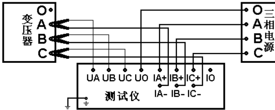
图 7-5 三相四线直接测量接线图
