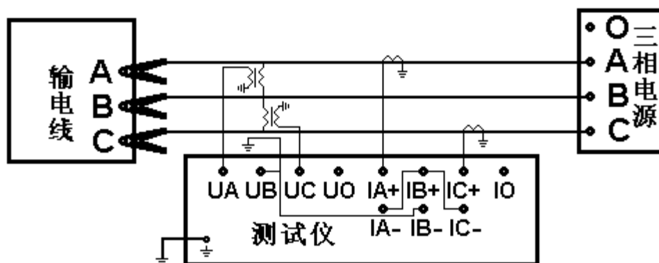
三相三线外接电压互感器和电流互感器接线
