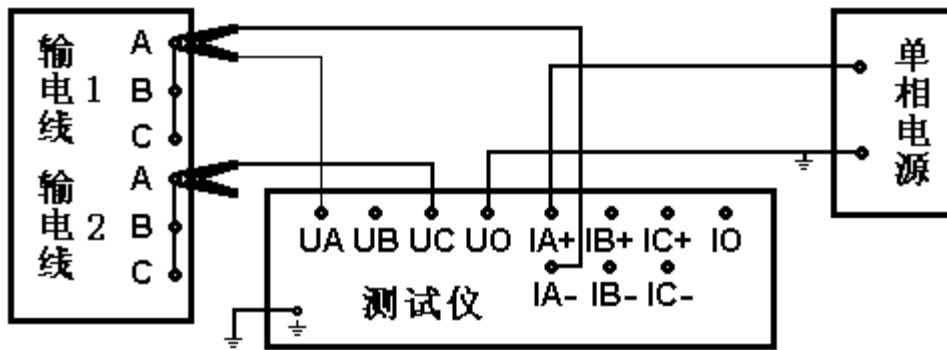
图 4-13 互感阻抗测量接线图
