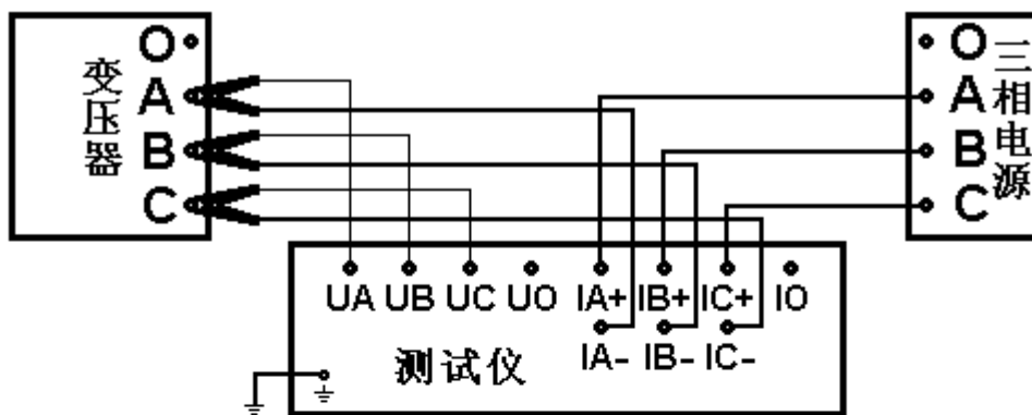
图 8-4 三相三线直接测量接线图
