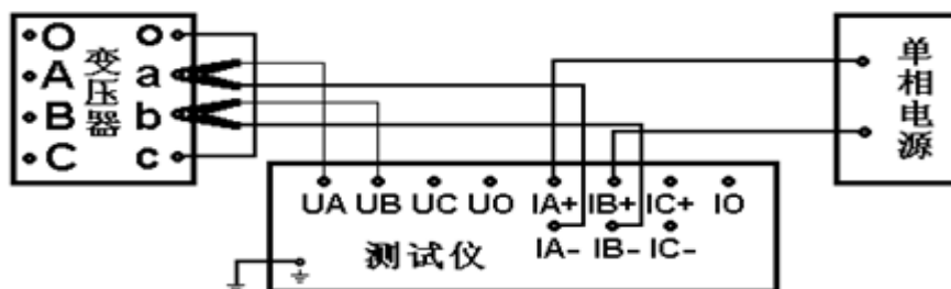
图 9-6 分相空载测量接线图
