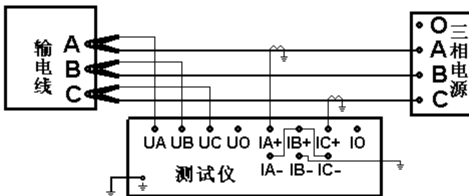
图 4-6 三相三线外接电流互感器接线图
