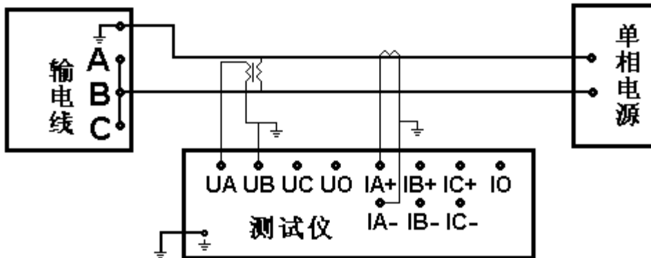
图 4-11 零序外接电压互感器和电流互感器接线图
