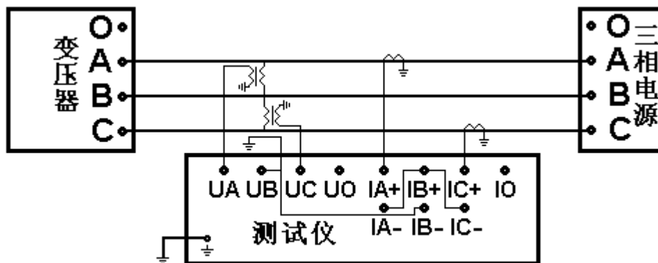
图 7-9 三相三线外接电压互感器和电流互感器接线
