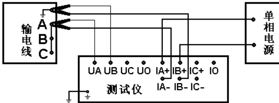
图 4-10 零序直接测量接线图
