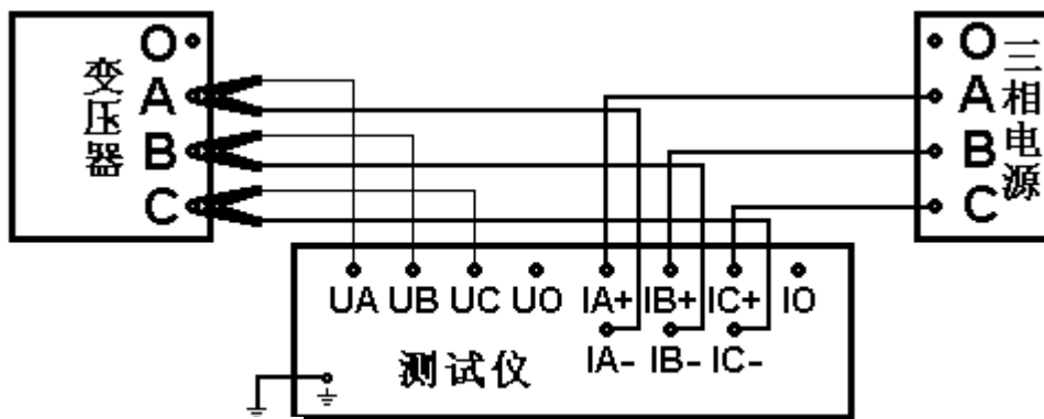
图 7-8 三相三线直接测量接线图
