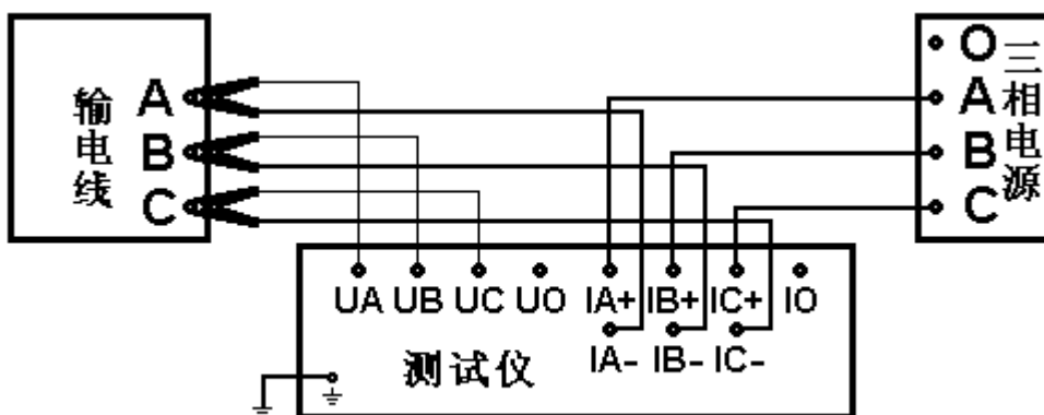
三相三线直接测量接线图
