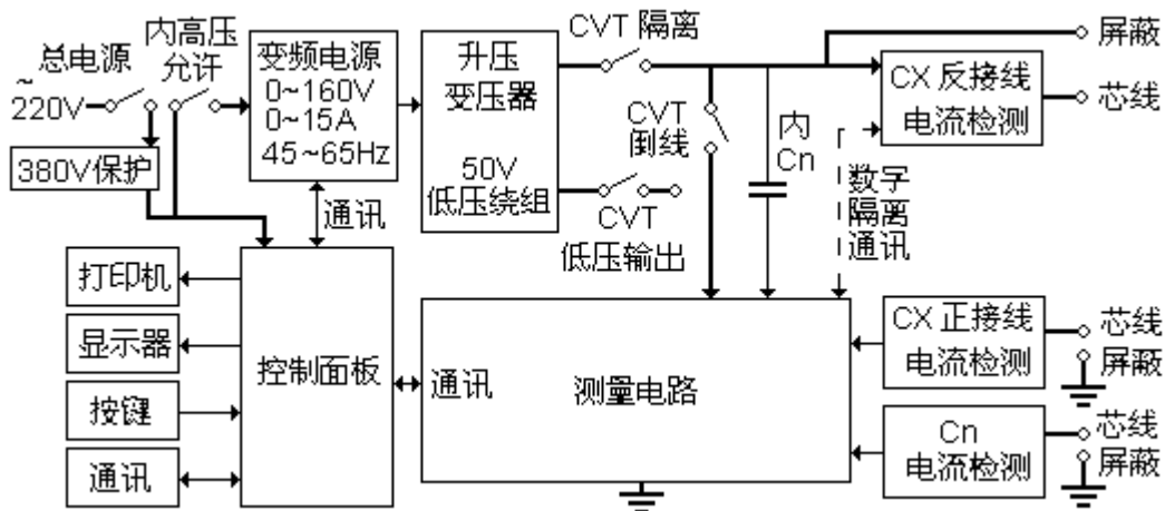
仪器结构框图
