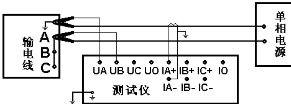
图 4-12 零序外接电流互感器接线图
