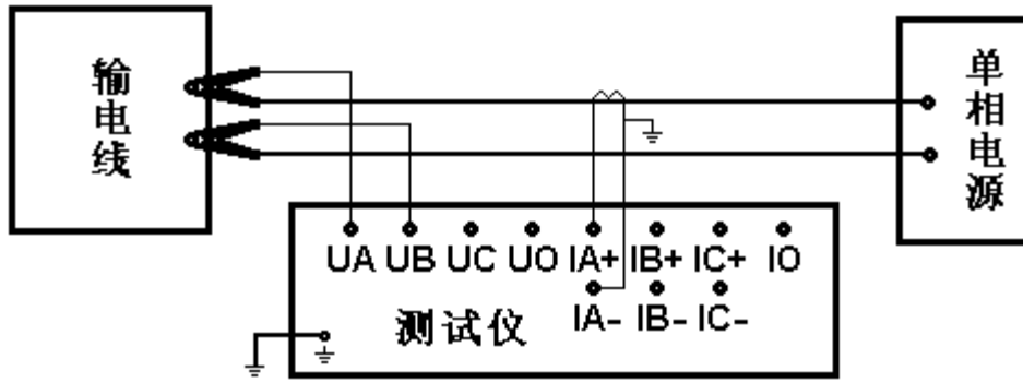
图 4-9 单相外接电流互感器接线图
