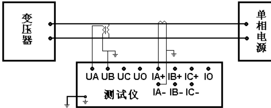
图 7-12 单相外接电压互感器和电流互感器接线图
