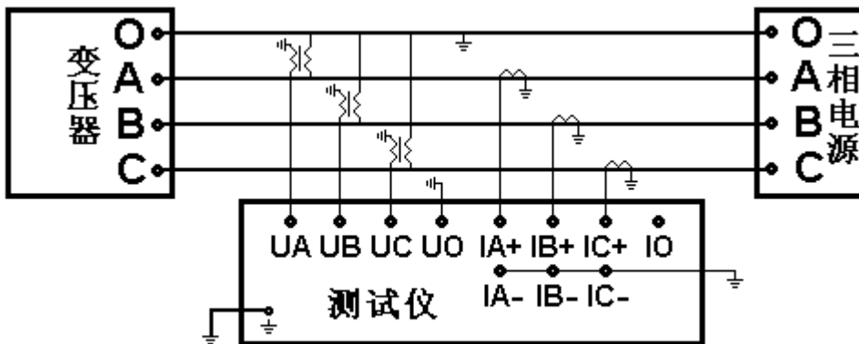
图 7-6 三相四线外接电压互感器和电流互感器接线图
