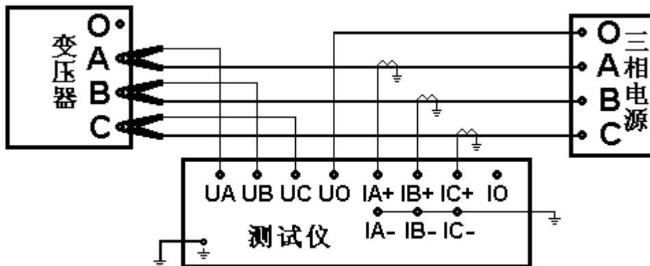
图 7-7 三相四线外接电流互感器接线图
